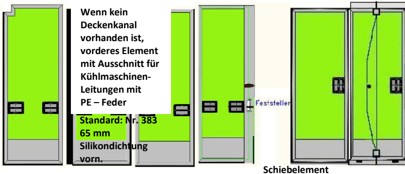
Typ 363 TYP 383 Typ 384 Typ 385 Typ384+Typ 364
